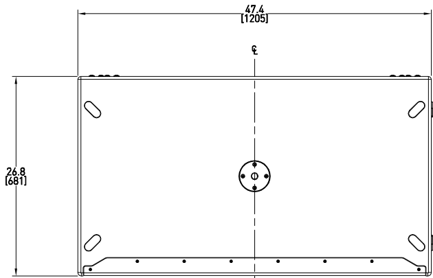
TOP
